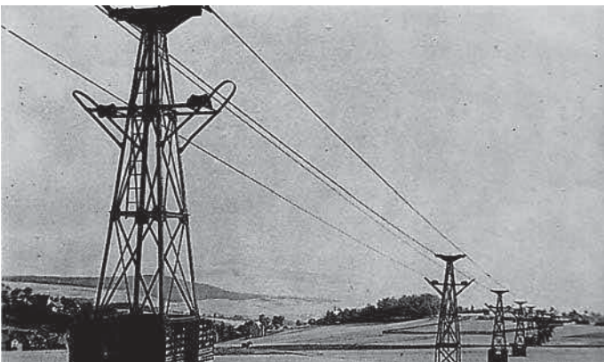
Die Seilbahn führte von der Be- und Entladestation Frankonia AG über die Frank- und Bernsbacher Straße, am Sportplatz vorbei zur Be- und Entladestation des Beierfelder Bahnhofs am Bahndamm.
